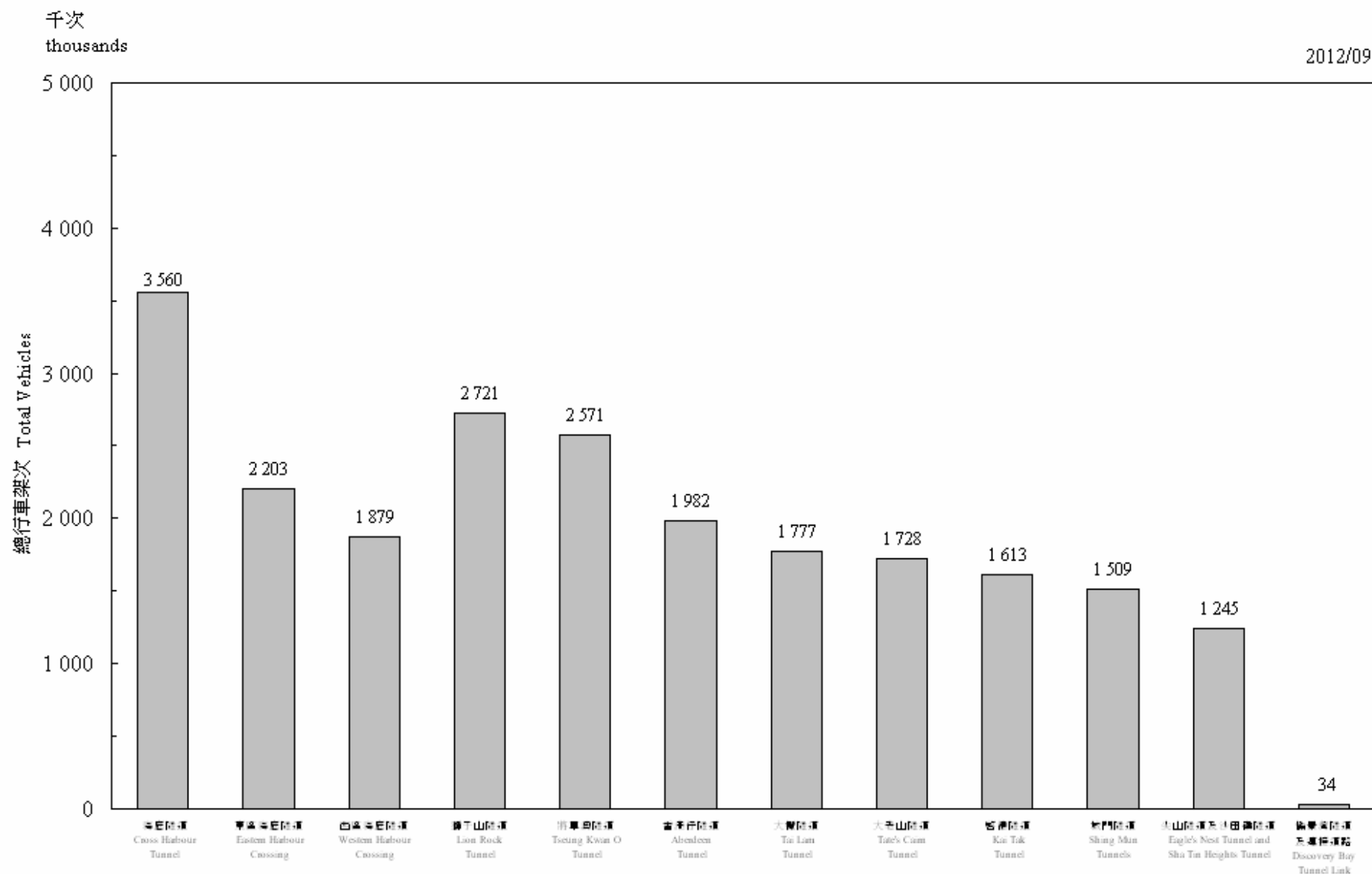
圖 3.1 - 隧道汽車流量 (二零一二年九月) Chart 3.1 - Vehicular Flow Through Tunnels (September 2012)
